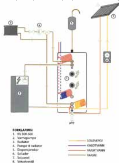
Eksempel: Solpanel, varmepumpe fast kondensering
