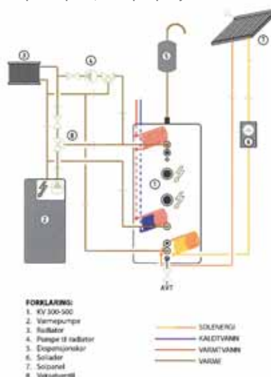
Eksempel: Solpanel, varmepumpe flytende kondensering
